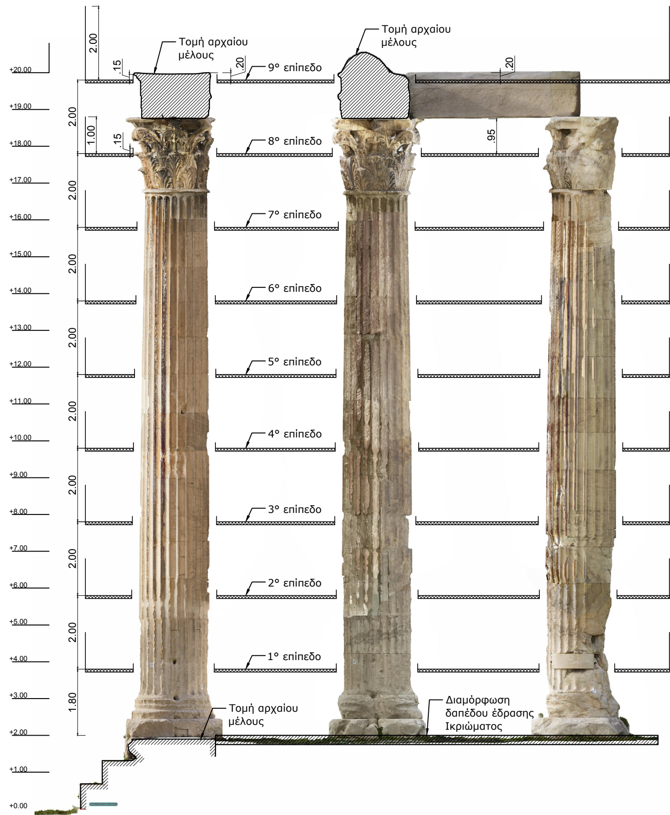
ΤΟΜΗ Α-Α
