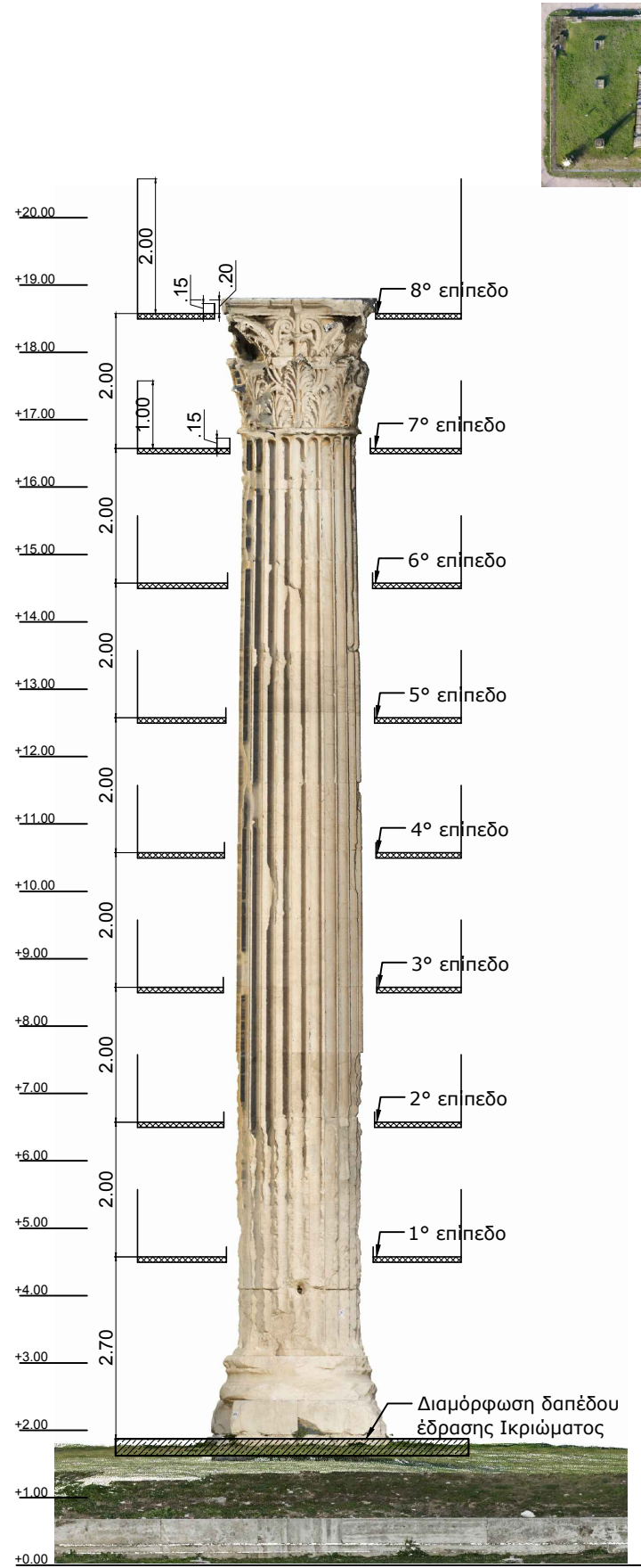
ΤΟΜΗ Β-Β
